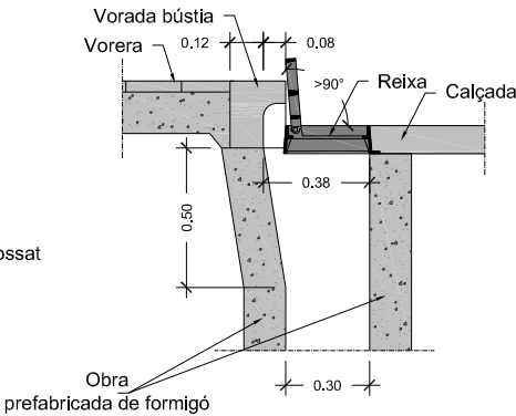
SECCIÓ TRANSVERSAL
