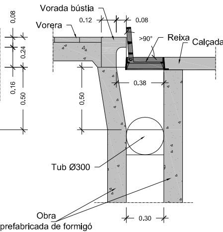
SECCIÓ TRANSVERSAL
