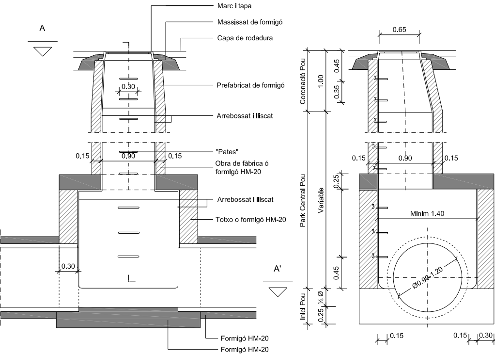
Secció b-b'
