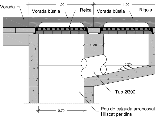
SECCIÓ LONGITUDINAL
