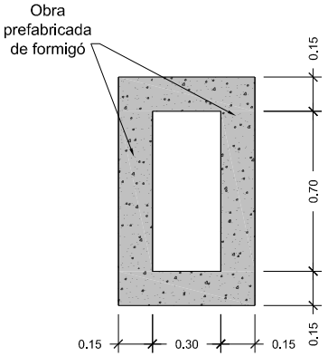
SECCIÓ POU DE CAIGUDA
