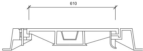
Secció A-A'
