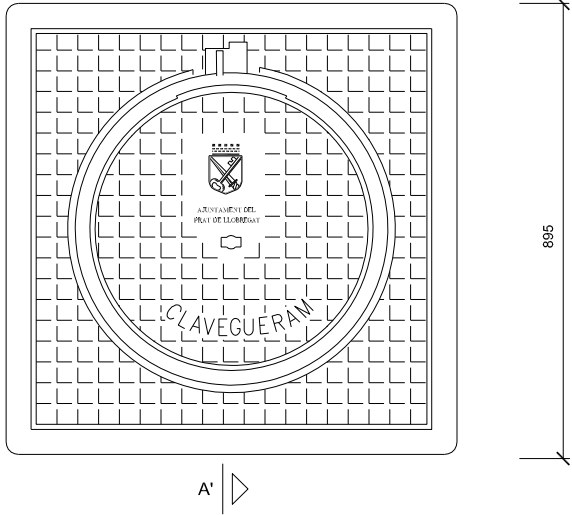
Tapa quadrada amb registre circular
