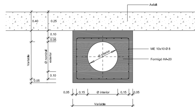
Secció protecció amb malla tub circular P.V.C. Escala 1/25
