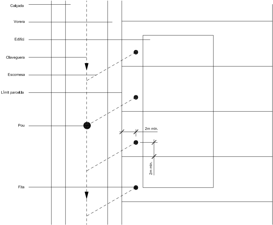
Esquema orientatiu Col·locació escomesa i fita en parcel·la Escala s/e
