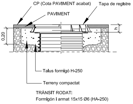
Detall colocació tapa
