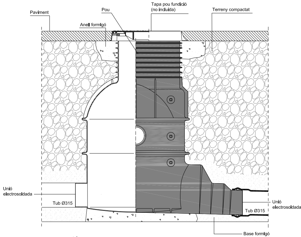
Alçat
