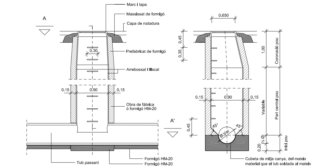
Secció b-b'
