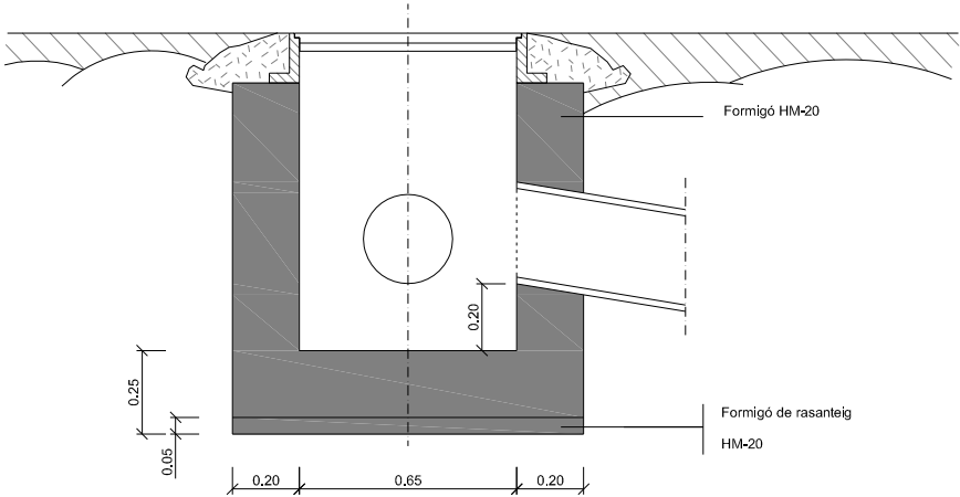
Secció A-A'
