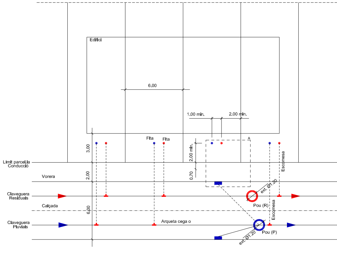
Planta Escala 1/250
