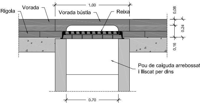
SECCIÓ LONGITUDINAL
