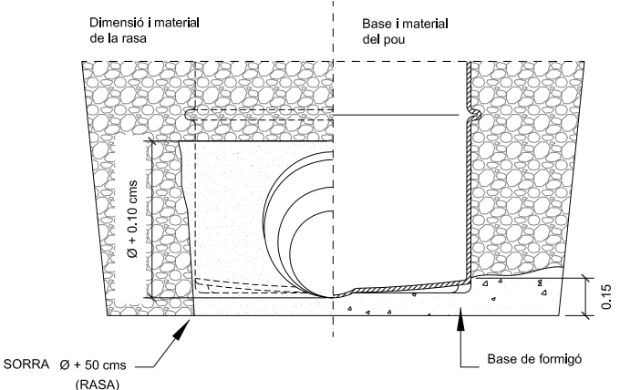
Detall colocació pou i rasa (cte-hs5)
