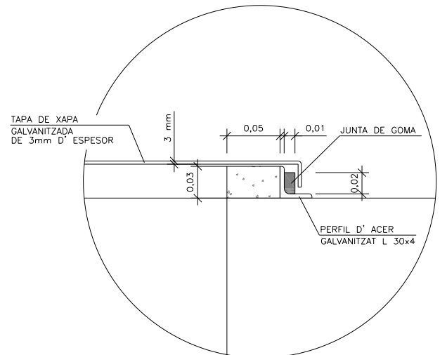
DETALL ESCALA 1/5
