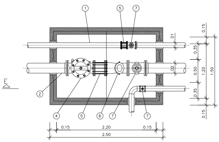
ARQUETA D' ENTRADA. PLANTA ESCALA 1/50
