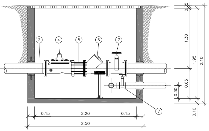
ARQUETA D' ENTRADA. SECCIÓ E-E' ESCALA 1/50
