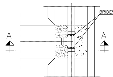
PLANTA DERIVACIÓ EN "T" ESCALA 1:25
