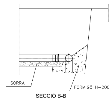
SECCIÓ B-B
