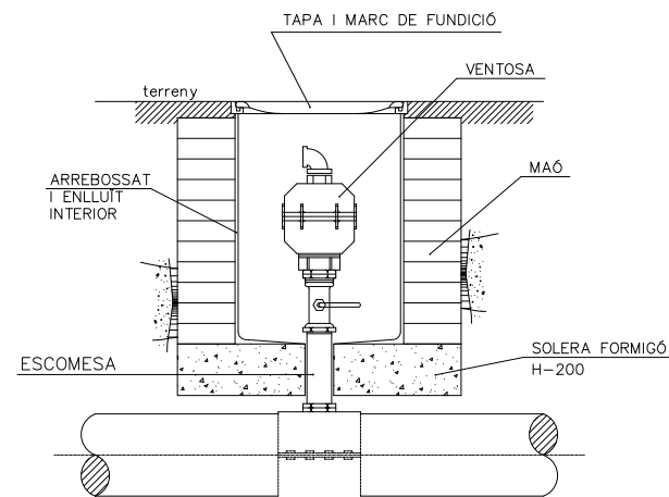
ARQUETA TIPUS PER A VENTOSA
