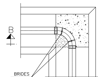
PLANTA DERIVACIÓ A 90° (COLZE) ESCALA 1:25
