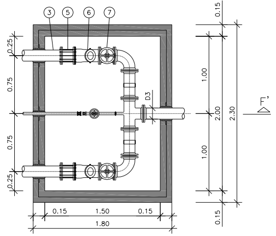
ARQUETA DE SORTIDA. PLANTA ESCALA 1/50
