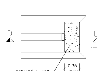
PLANTA BRIDA CEGA ESCALA 1:25
