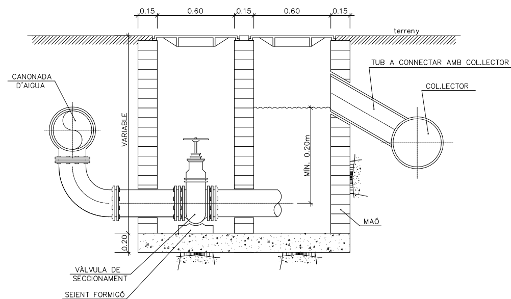
TAPA I MARC DE FUNDICIÓ Tapa 40x40 per a canonades fins Ø100 Tapa 60x60 per a canonades ≥ Ø150 ARQUETA TIPUS PER A DESCÀRREGA ESCALA 1:10
