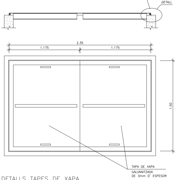
DETALLS TAPES DE XAPA ESCALA 1/30
