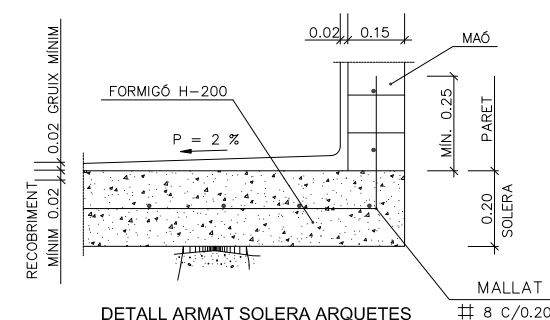
DETALL ARMAT SOLERA ARQUETES PER A ARQUETES DE LLUM A PARTIR DE 0.60m ESCALA 1:10
