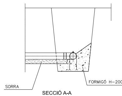
SECCIÓ A-A
