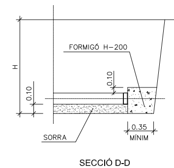
SECCIÓ D-D
