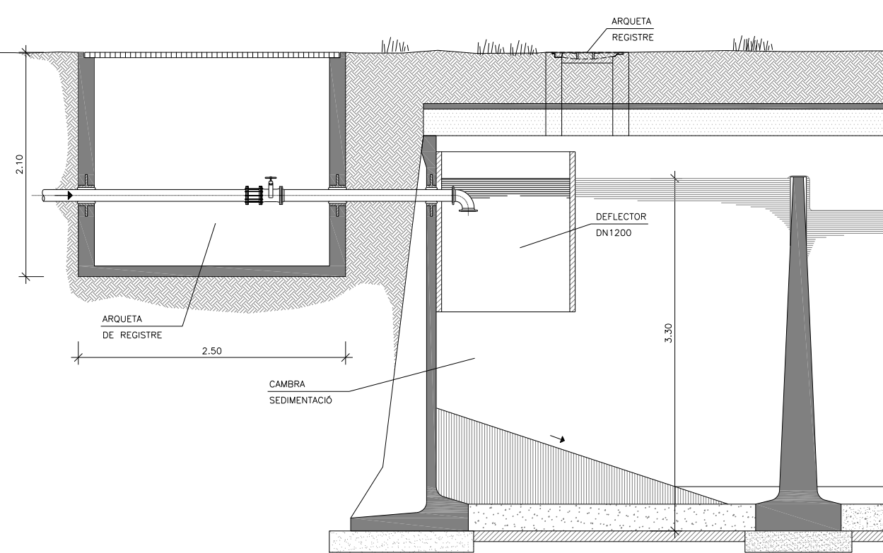
CAMBRA SEDIMENTACIÓ. SECCIÓ D-D' ESCALA 1/50
