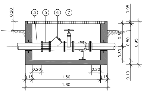
ARQUETA DE SORTIDA. SECCIÓ F-F' ESCALA 1/50
