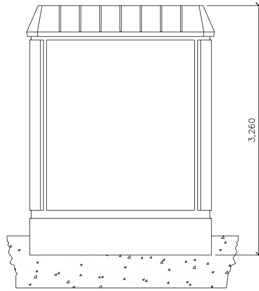
OBRA CIVIL ESTACIÓ TRANSFORMADORA LATERAL ESQUERRE ESCALA: 1/50
