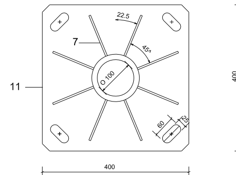
DETALL PLANTA PLACA 1/10
