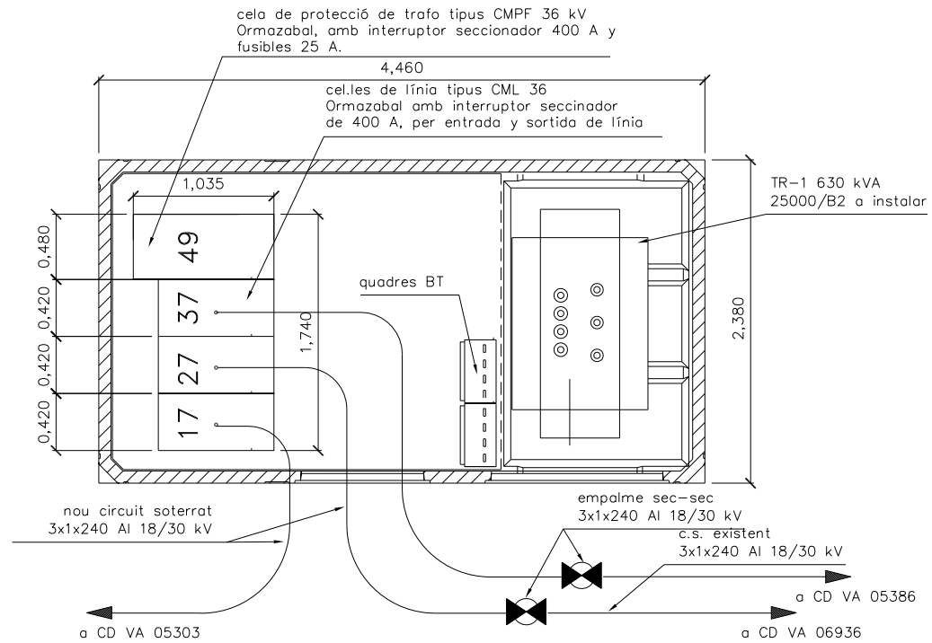
OBRA CIVIL ESTACIÓ TRANSFORMADORA PLANTA PFU4 ESCALA: 1/50
