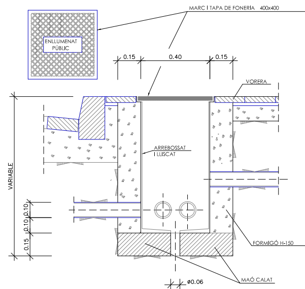
TRONETA TIPUS Escala 1/25 (cotes en m.)
