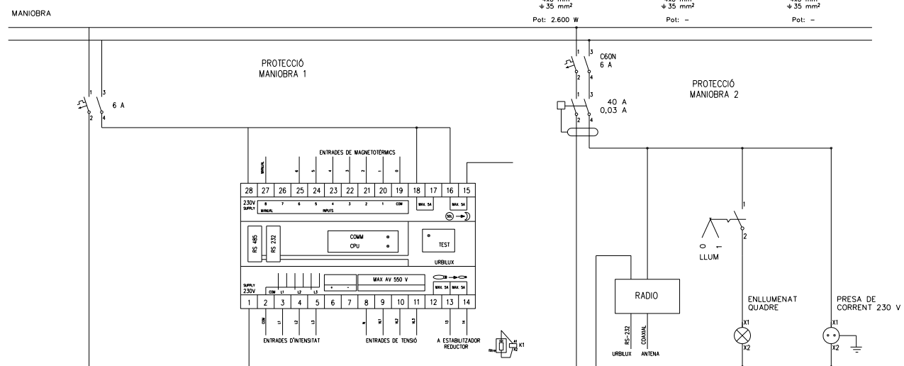
QUADRE ELÈCTRIC D'ENLLUMENAT - ESQUEMA DE MANIOBRA
