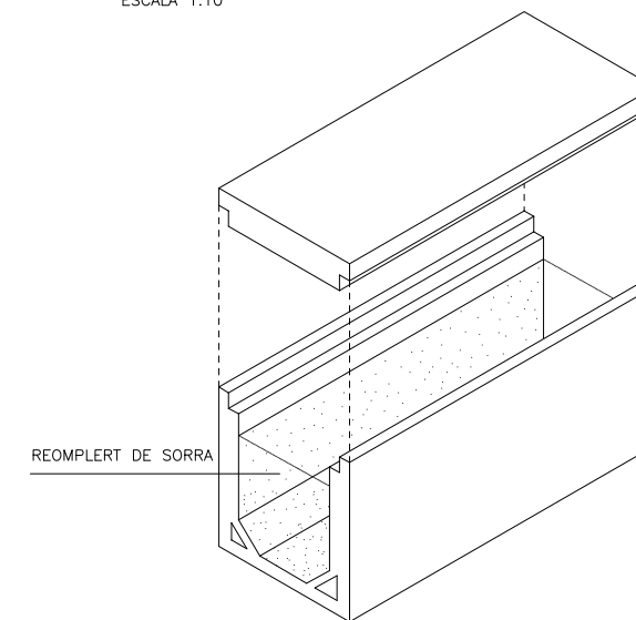
DETALL CANALETA CERÀMICA
