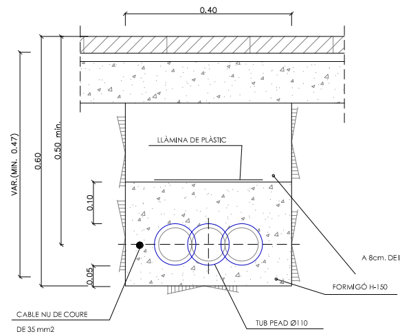
RASA TIPUS PER A ENTUBAR CABLES A ZONA DE VORERES Escala 1/12.5 (cotes en m.)
