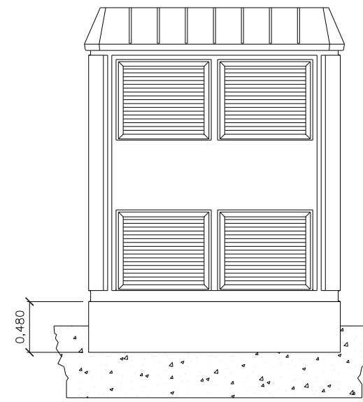
OBRA CIVIL ESTACIÓ TRANSFORMADORA LATERAL DRET ESCALA: 1/50
