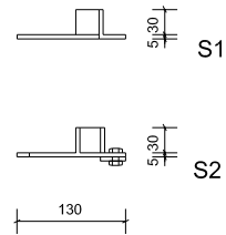
SECCIONS BRAÇ DE SUPORT 1/10
