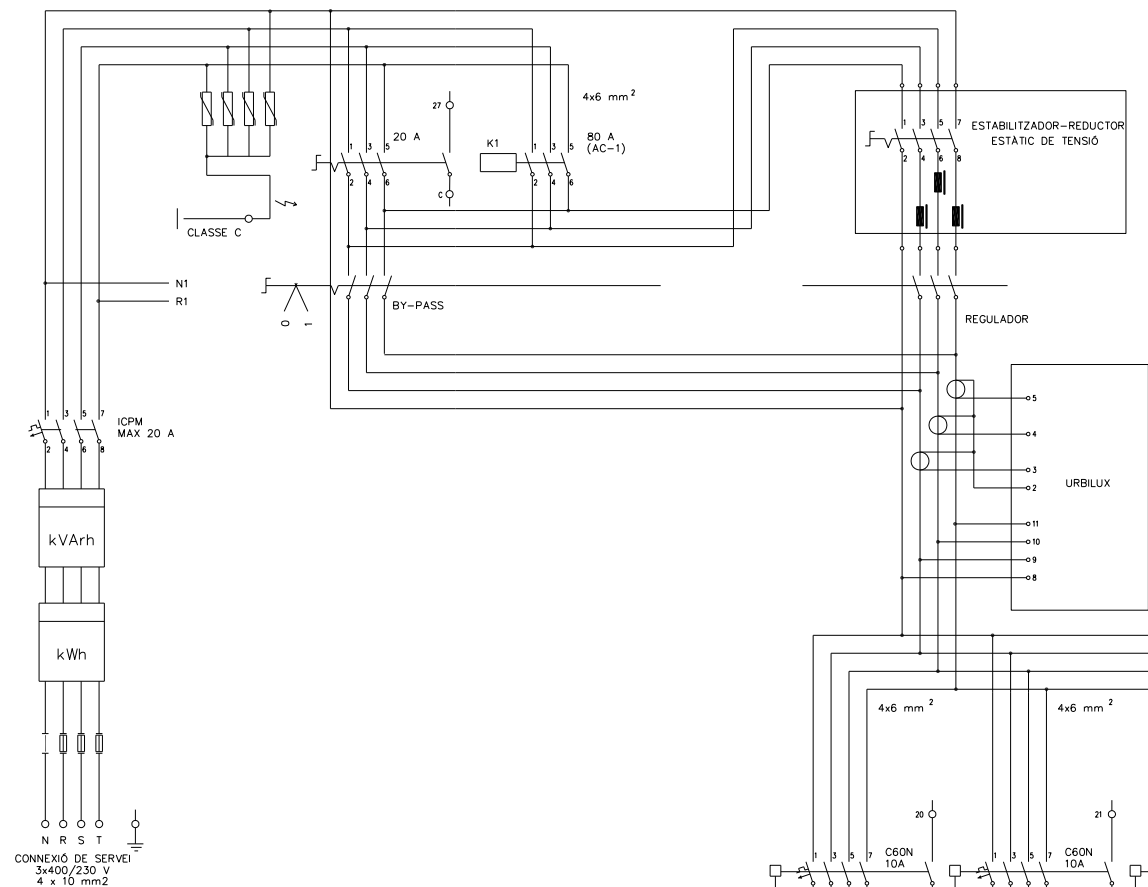
QUADRE ELÈCTRIC D'ENLLUMENAT - ESQUEMA DE POTÈNCIA
