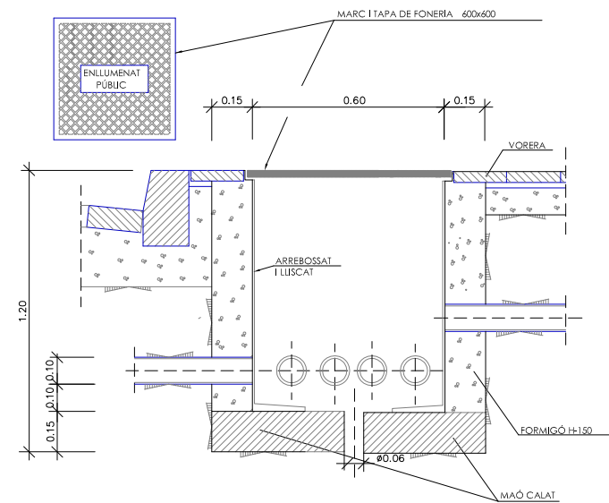
TRONETA PER QUADRE D'ENLLUMENAT I ENCREUAMENT DE CALÇADES Escala 1/25 (cotes en m.)
