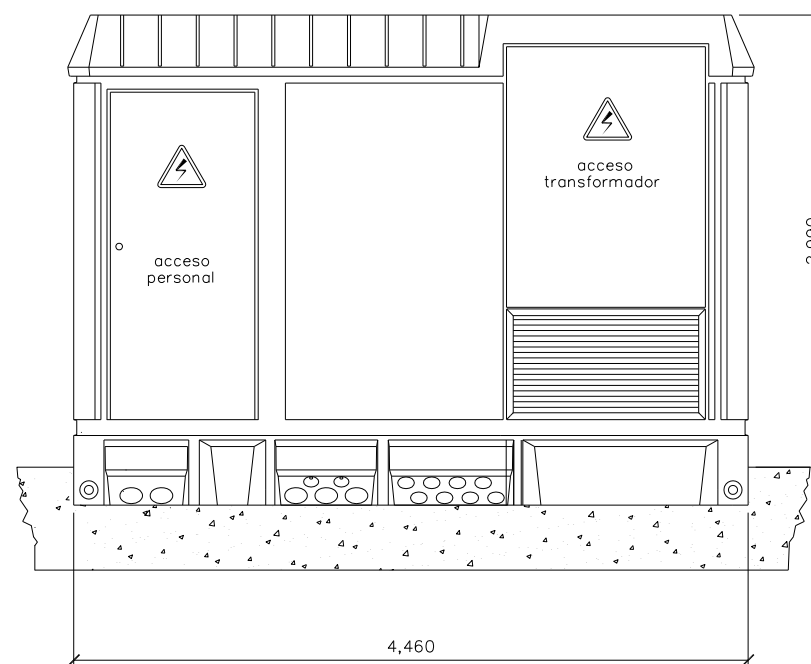
OBRA CIVIL ESTACIÓ TRANSFORMADORA ALÇAT FRONTAL ESCALA: 1/50
