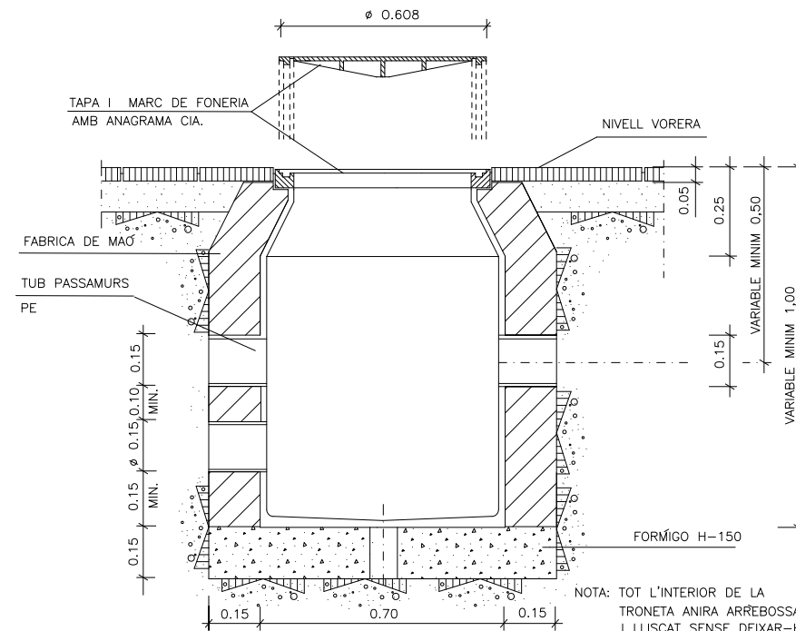
SECCIO A-A
