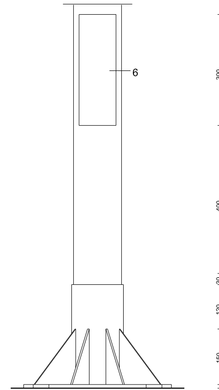
DETALL ALÇAT PLACA 1/10
