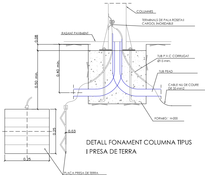
FONAMENTS DE LES COLUMNES
