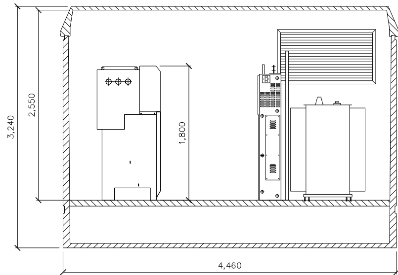
OBRA CIVIL ESTACIÓ TRANSFORMADORA SECCIÓ PFU4 ESCALA: 1/50
