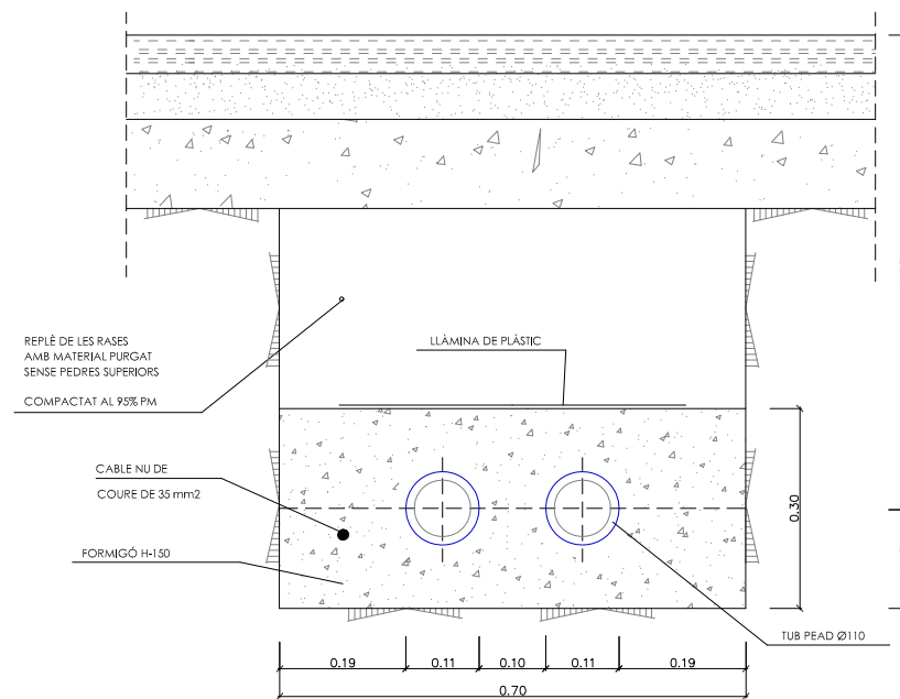
RASA TIPUS PER A ENTUBAR CABLES A ZONA DE VIALS Escala 1/12.5 (cotes en m.)
