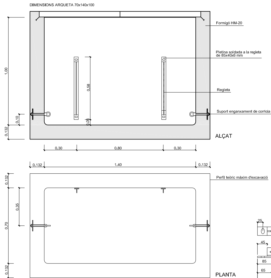
Arqueta prefabricada 70x140x100 en vorera ESCALA 1:20
