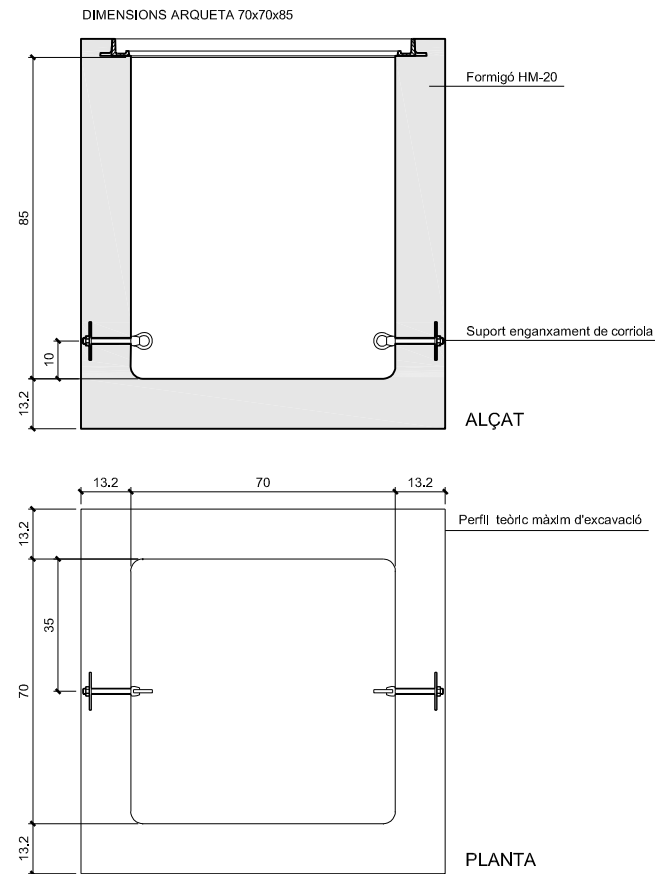
Arqueta prefabricada 70x70x85 en vorera ESCALA 1:20
