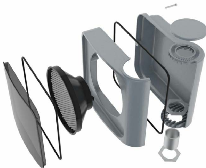
Imatge 4 DETALL MONTATGE ÒPTICA LED
